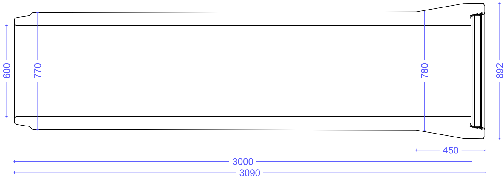
Standaard buis
