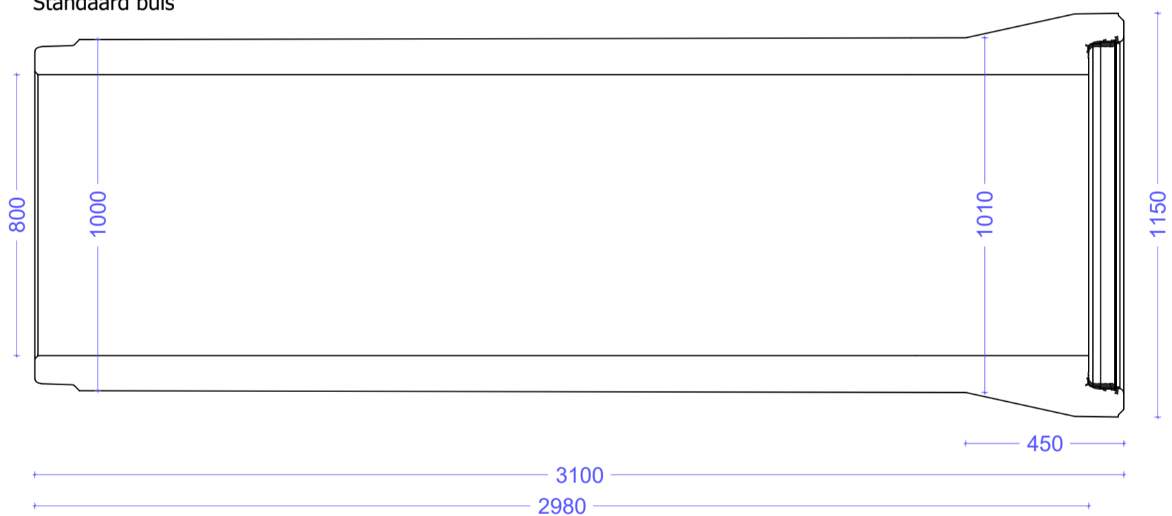
Standaard buis
