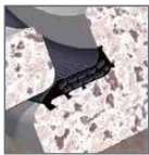
Beginsituatie glipdichting 1e phase de l'emboîtement
