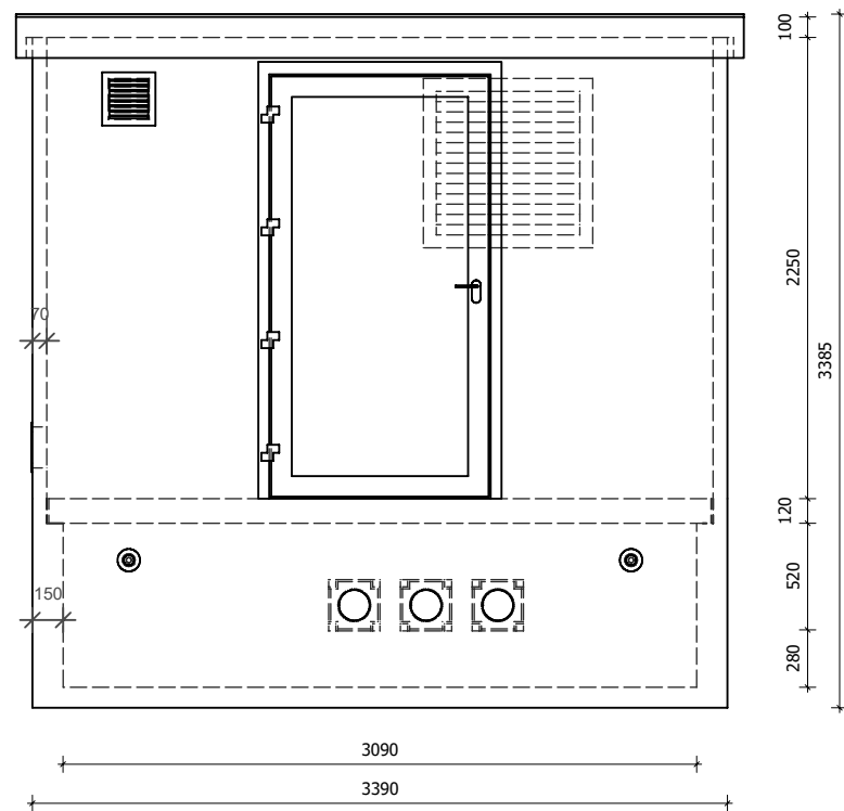
Vooraanzicht
