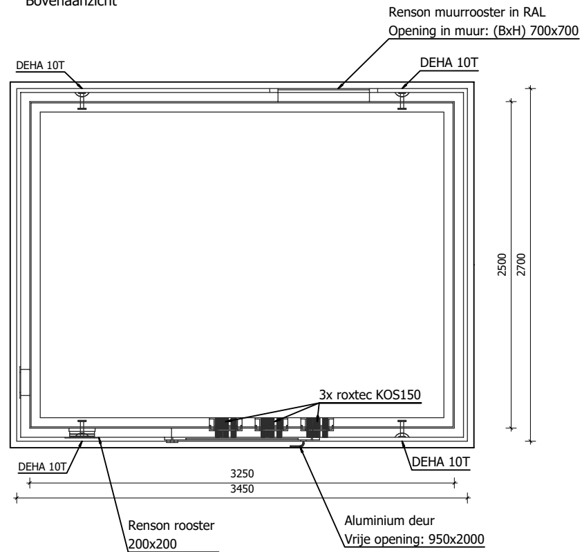
Bovenaanzicht
