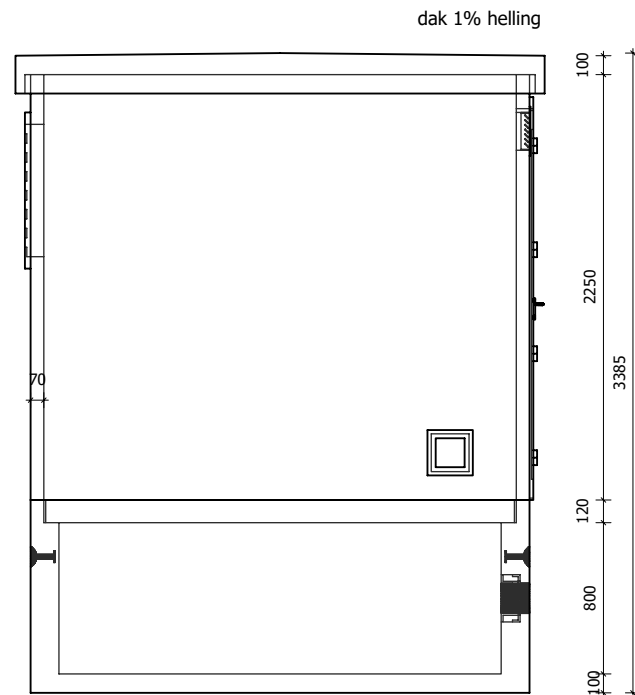
Linkerzij aanzicht
