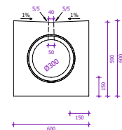
Doorsnede Coupe
